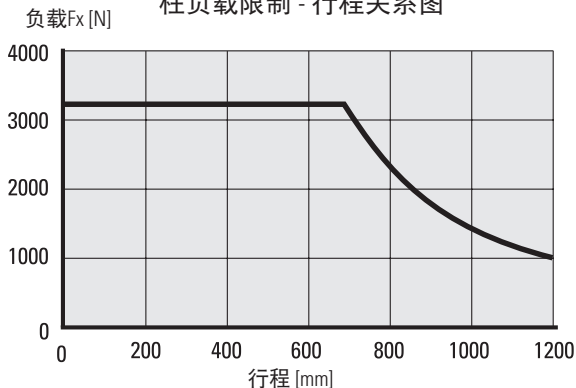
柱负载限制 - 行程关系图
