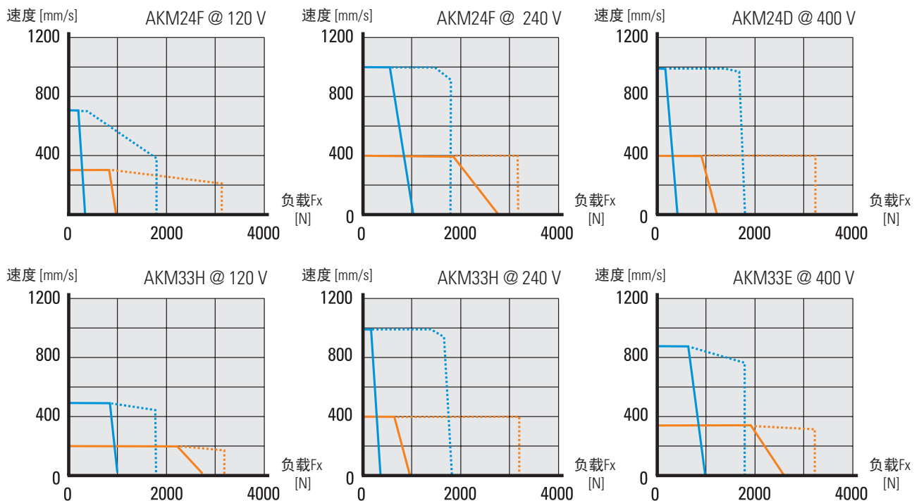
带平行安装AKM伺服电机的PC32
