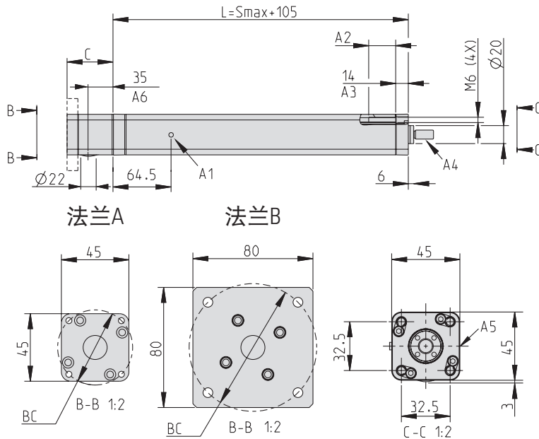
配有RediMount法兰的直线型执行器尺寸
