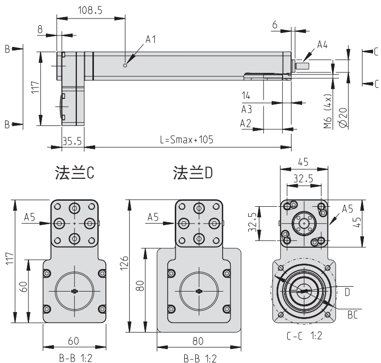
配有RediMount电机安装法兰的平行型执行器尺寸
