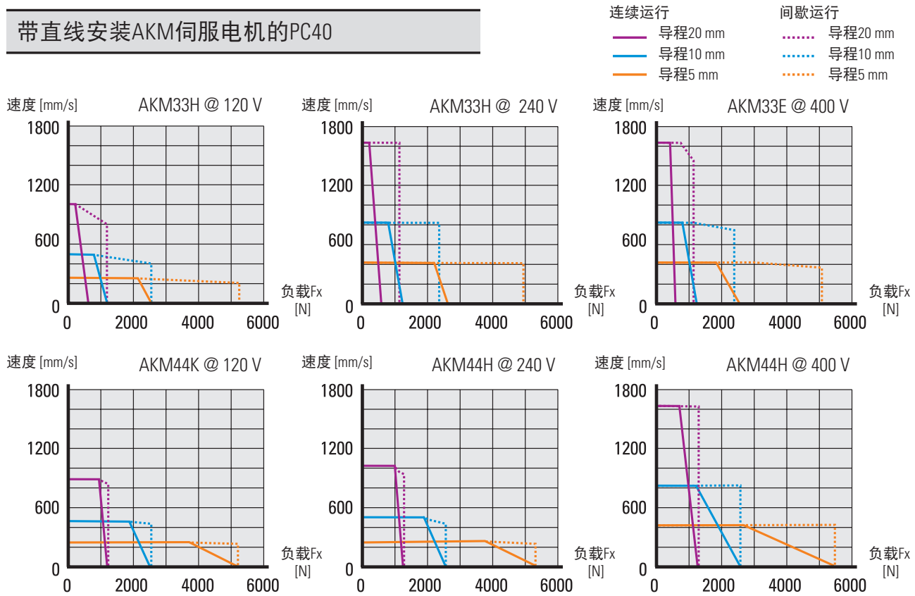
带平行安装AKM伺服电机的PC40
