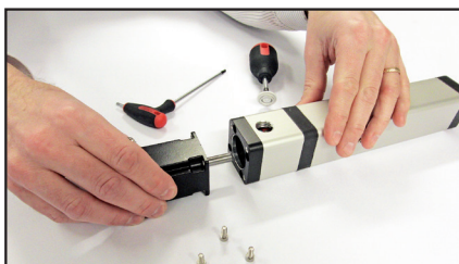
将电机轴插入联轴器内
