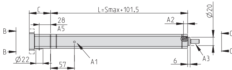
配有RediMount法兰的直线型执行器尺寸
