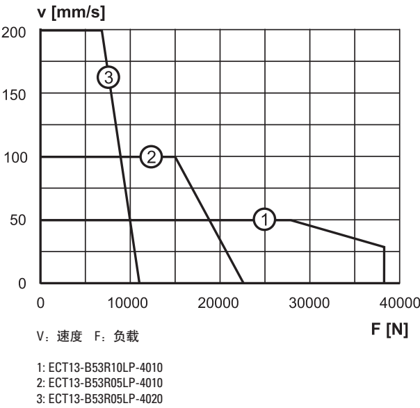
速度与负载
