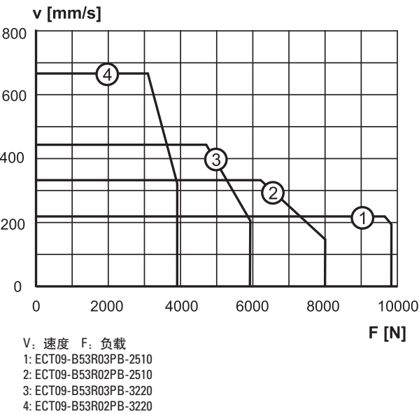
速度与负载
