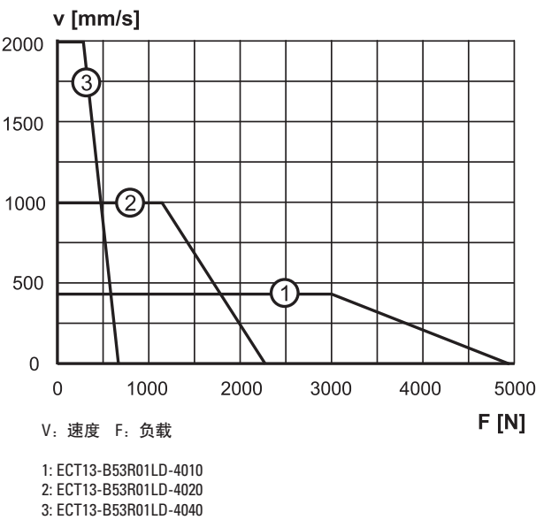
速度与负载
