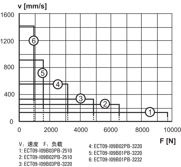
速度与负载
