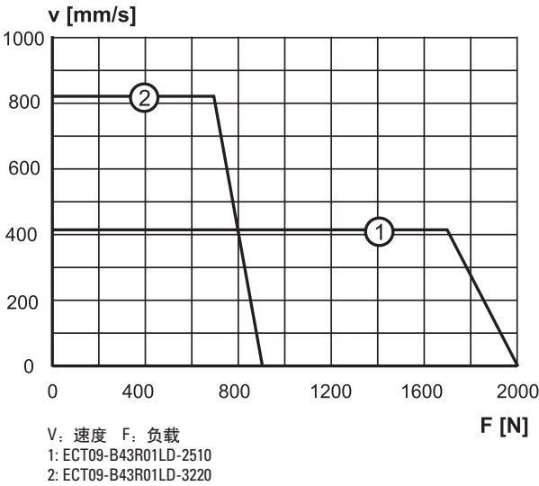
速度与负载
