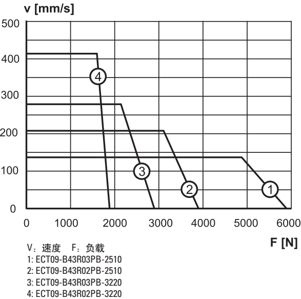
速度与负载
