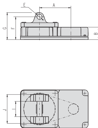
BGM81 – R型U形夹选件
