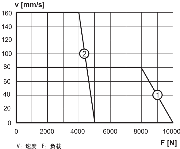
速度与负载
