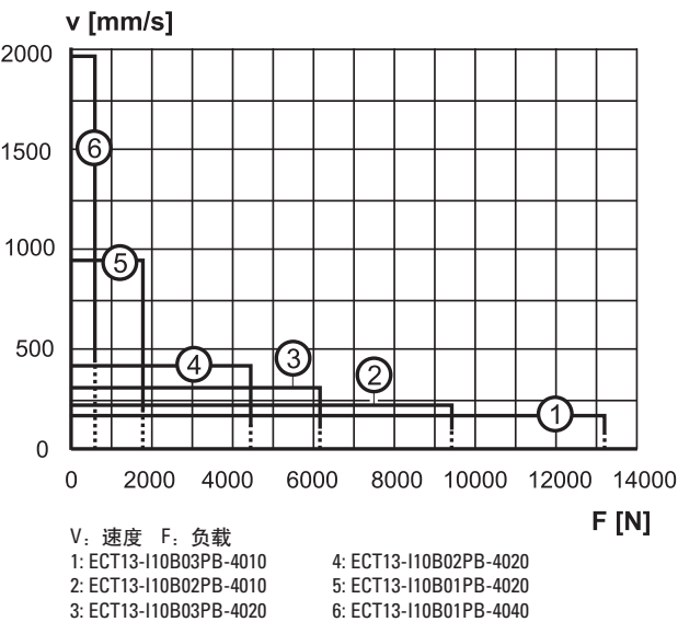
速度与负载
