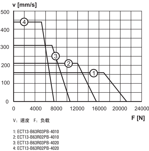
速度与负载
