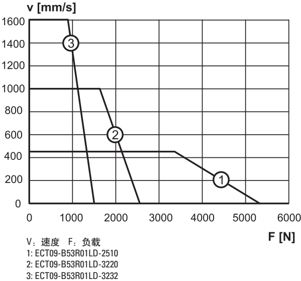
速度与负载
