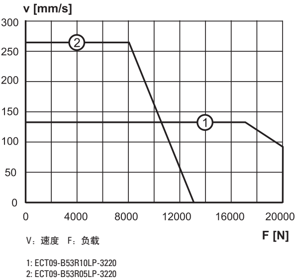
速度与负载
