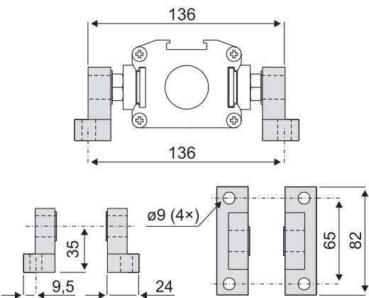
T60用耳轴支架套件
