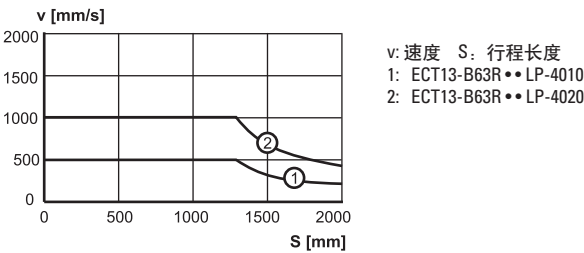
界速度与行程
