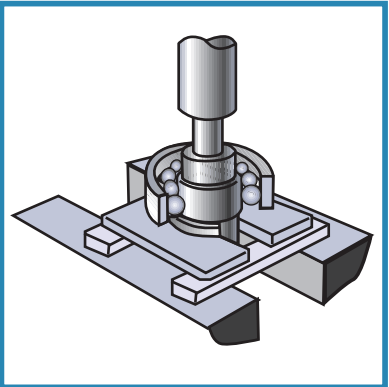
图4.3 用压力机，注意垫块 Fig.4.3 Use Press & Pad
