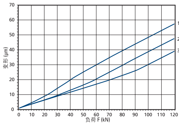
65 压缩负荷，预负荷 1、2、3
