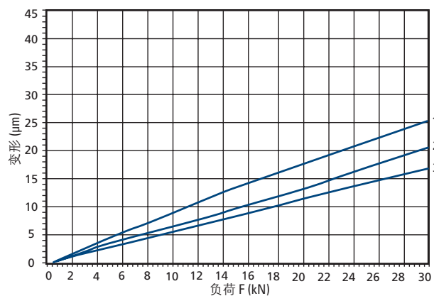
35 压缩负荷，预负荷 1、2、3
