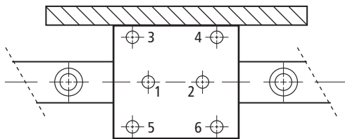
图 7 建议的坚固顺序
