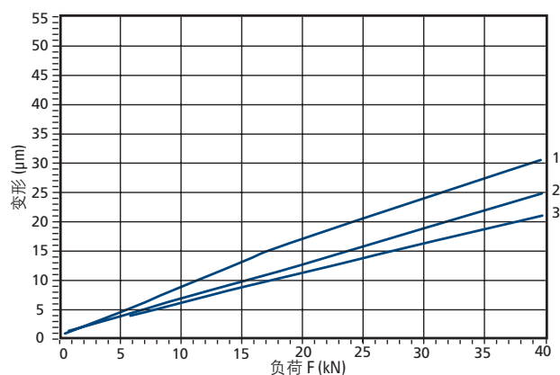
45 压缩负荷，预负荷 1、2、3
