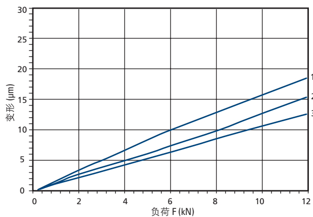
25 压缩负荷, 预负荷 1、2、3
