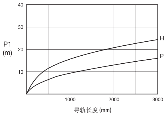
图 2 - 平行度
