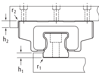
图 5 肩部高度和圆角半径
