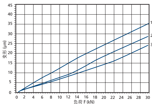
35 压缩负荷，预负荷 1、2、3
