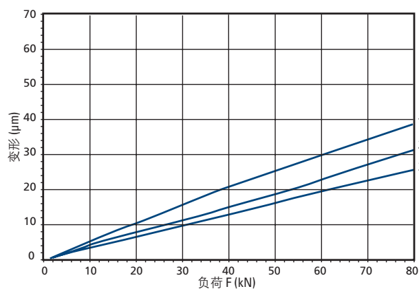
55 压缩负荷, 预负荷 1、2、3
