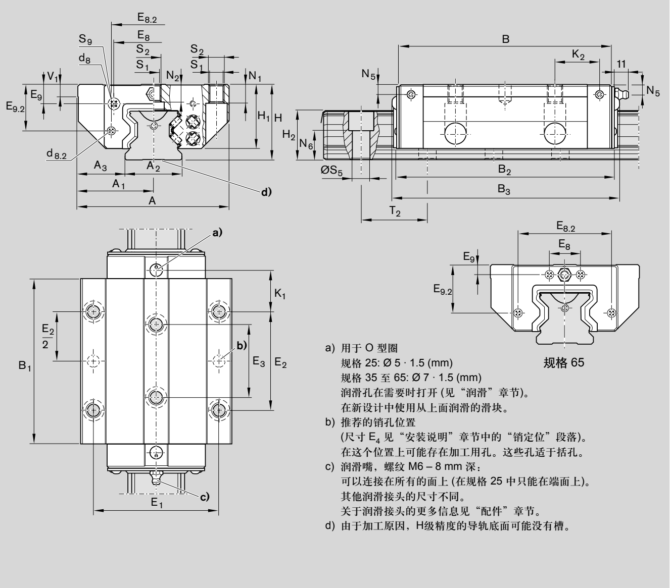
标准滑块 FLS R1853 ... 10
