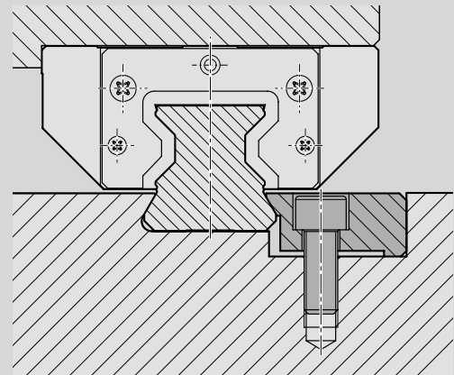
带 V 形导轨的滚柱导轨导向系统
