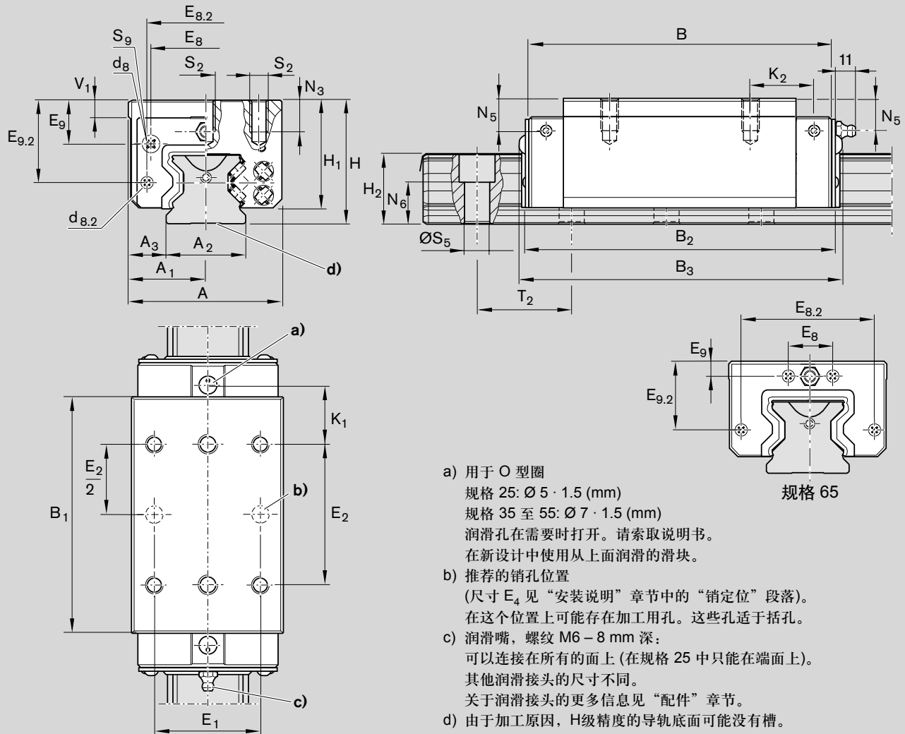
标准滑块 SLH R1824 ... 10
