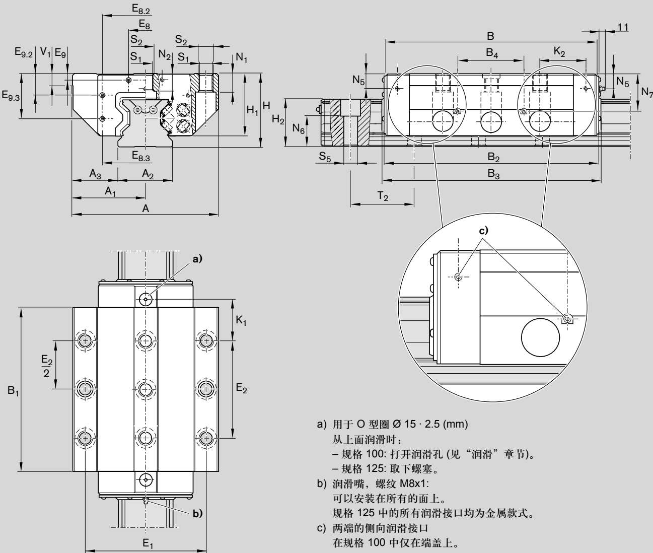
重载滑块 FLS R1863 ... 10 和 FLS R1863 ... 60
