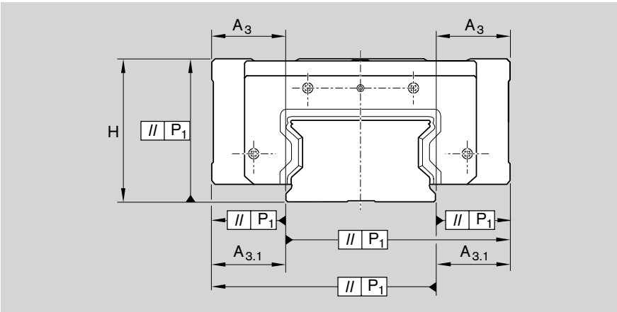
钢制宽滚柱导轨导向系统
