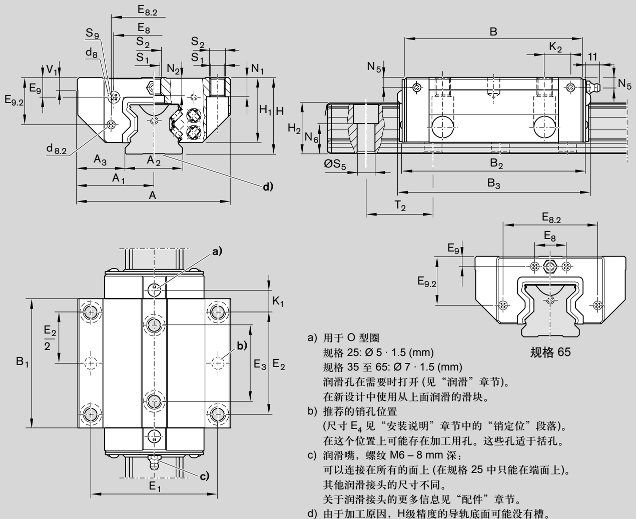
标准滑块 FNS R1851 ... 10
