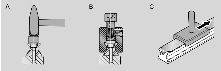
在导轨上安装孔盖或防护带
