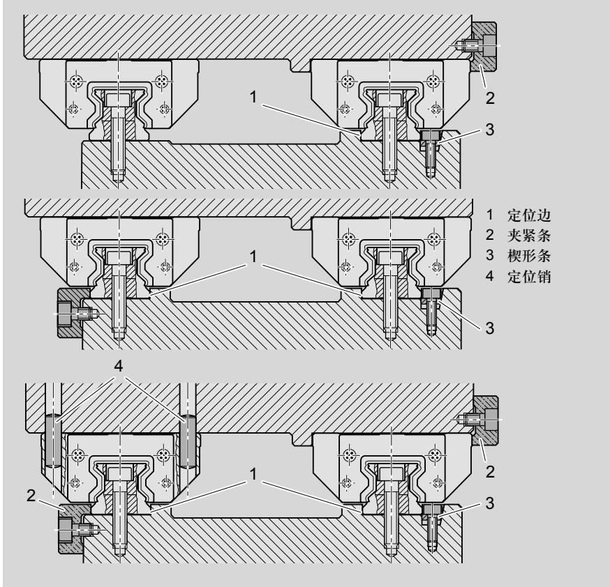
导轨和/或滑块的侧向固定 (举例)
