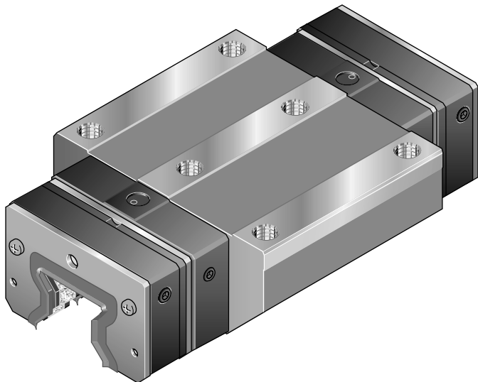
带两个前置润滑单元和前置密封的标准滑块
