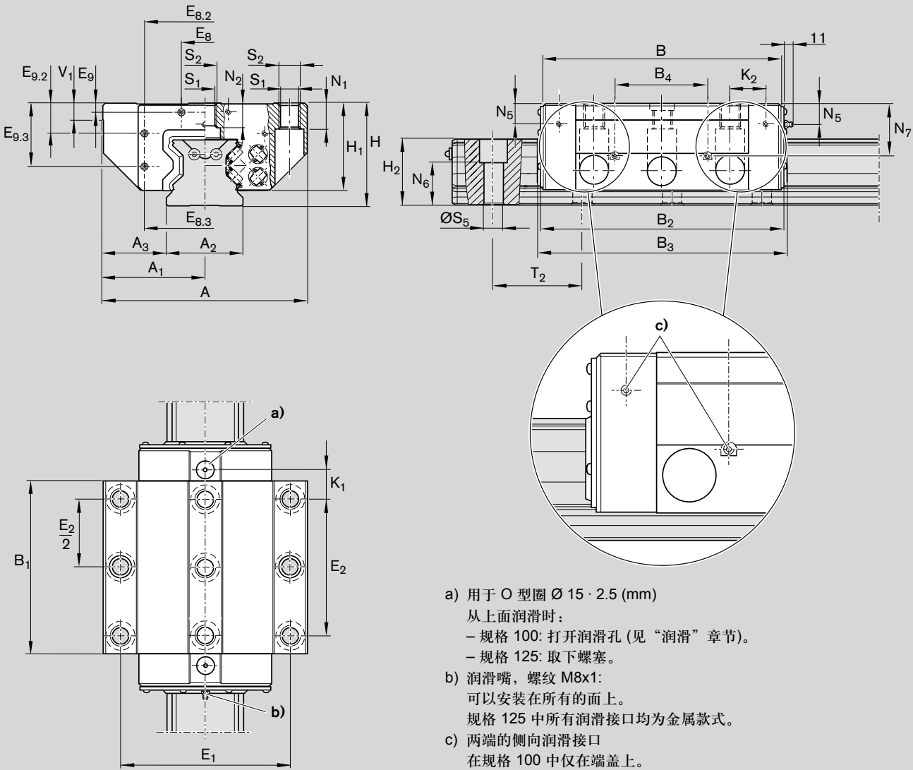
重载滑块 FNS R1861 ... 10 和 FNS R1861 ... 60
