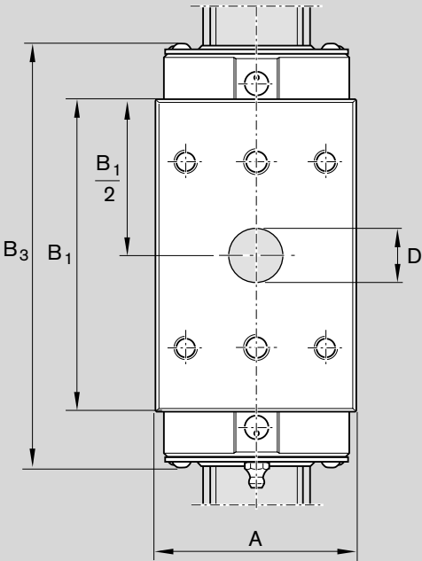
安装滑块 SLH R1829
