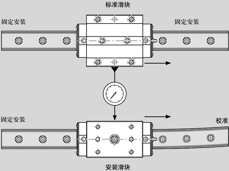
用安装滑块进行安装
