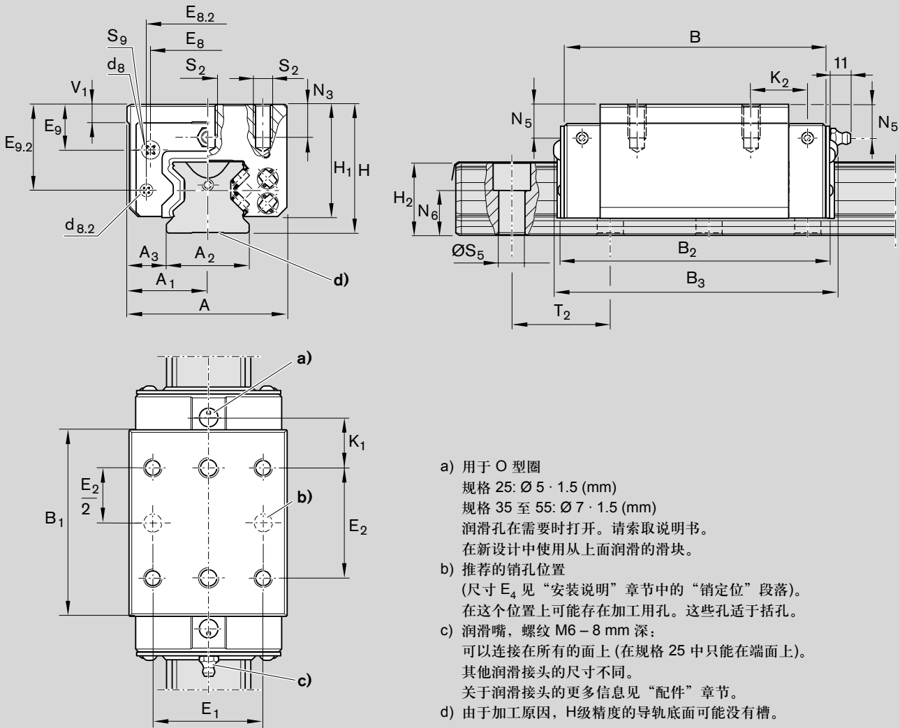
标准滑块 SNH R1821 ... 10
