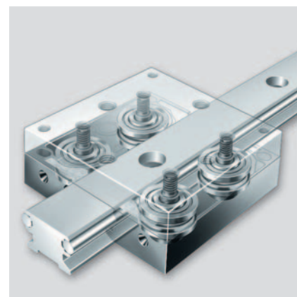
速度达到10 m/s：轻量化设计的滚轮直线导引系统
