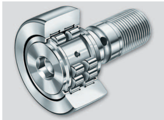
加大的储脂槽降低维护成本：重载用螺栓型滚轮PWKR
