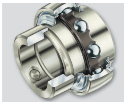
带Corrotect®涂层的防腐蚀外球面球轴承
