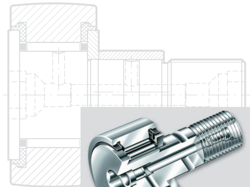
外圈表面和支承轨道无磨损：INA带Triondur 涂层支承型滚轮，用于PET瓶灌装机星轮传输单元的凸轮控制系统中（图片：KRONES）。
