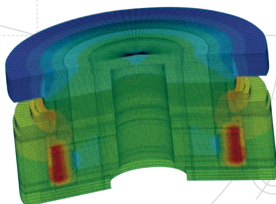
较低的轴承温度有效的保证了机床精度
