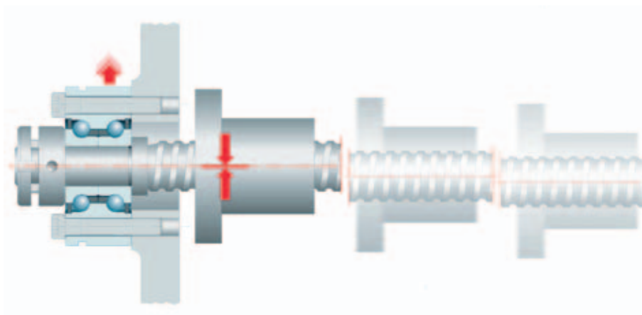
通过调节丝杠驱动螺母实现轴承的对中
